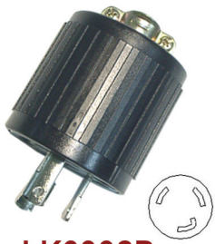
LK6332B 3P30A250V NEMA L6-30P
