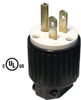
LK7515P 15A 125V NEMA 5-15P
