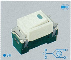
WNF5152 螢光開關C(3路) 15A 110V AC用
