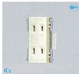
WNF1402 埋入瞬間雙插座 15A 125V AC
