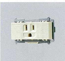
WNF11016 埋入式5.5mm 2 絞線用附接地極插座 15A 125V AC
