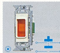
WN4500-8 緊急用埋入式押釦 6A 300V AC
