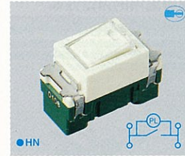
WNF5051 螢光開關B(單切)(附標名) 15A 110V AC用
