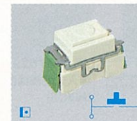
WN5401K-8 押釦(單切) 10A 300V AC
