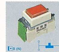
WN5460K-8 標名押釦B(B接點) 10A 300V AC ※可以表示負荷名
