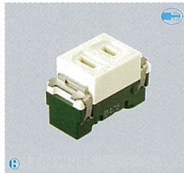
WNF1001 埋入插座 15A 125V AC
