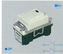
WN5003-802 開關D(兩切) 15A 300V AC
