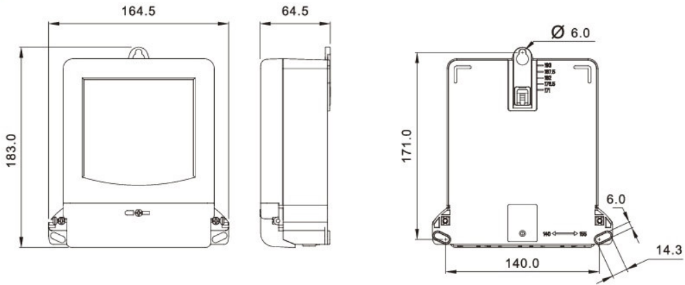
【固定孔位置圖】
