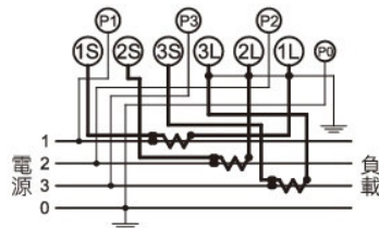
BAW-4C 三相四線式
