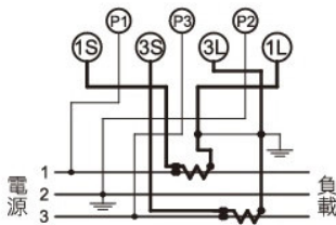
BAW-3C 三相三線式
