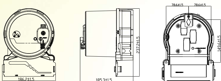
單相三線接法：2接中性線
